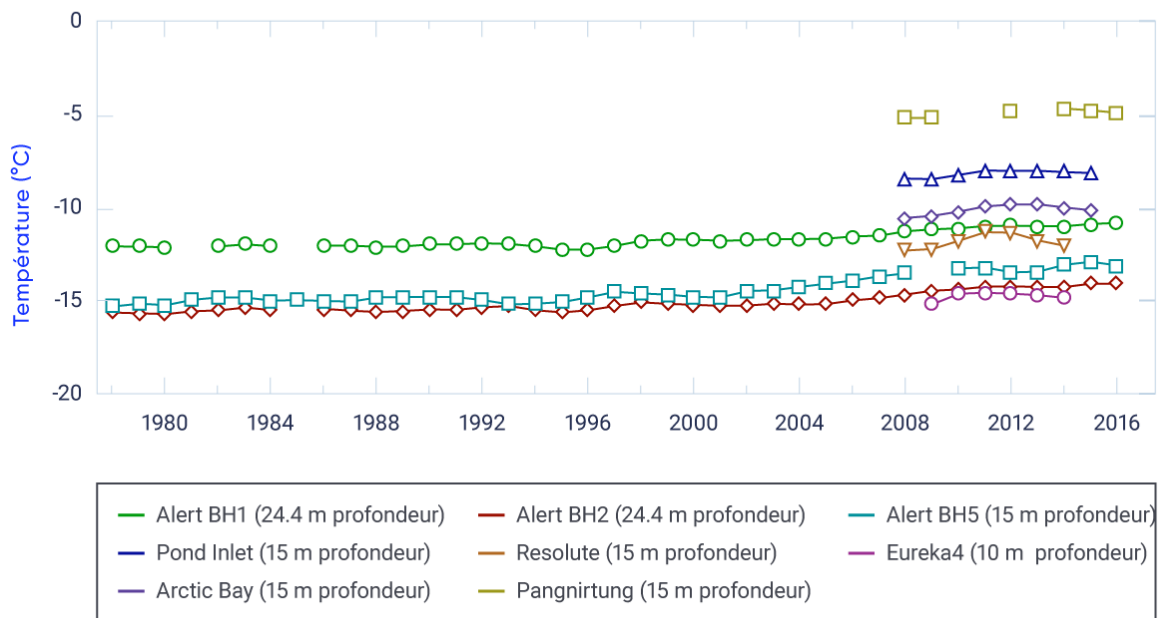
Figure 5.17: Tendances des températures du pergélisol
