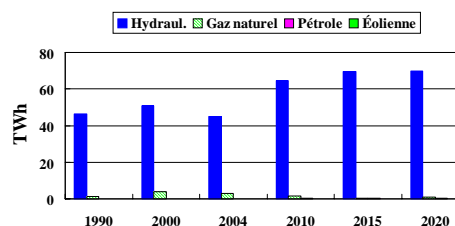
Figure BC5 Production d'électricité
