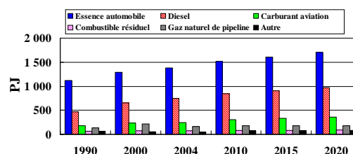
Figure T1 Demande énergétique d'utilisation finale selon le type de carburant Secteur des transports
