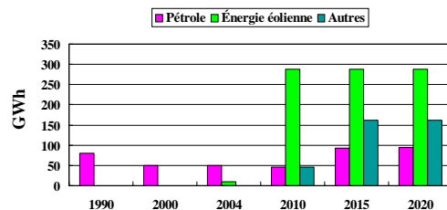
Figure IPE4 Production d'électricité
