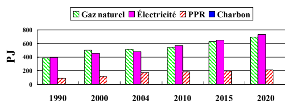
Figure C1 Demande énergétique d'utilisation finale selon le type d'énergie Secteur commercial
