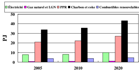
Figure IN3 Demande énergétique d'utilisation finale selon le type d'énergie Ciment
