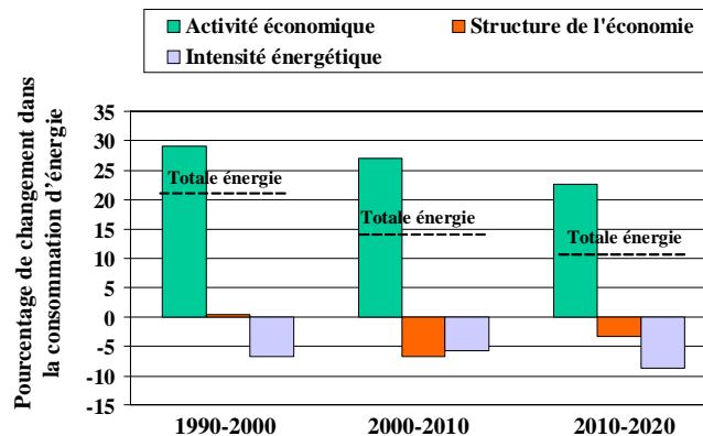
Figure PR2 Facteurs des changements dans l'utilisation énergétique—Biens et Services (1990-2020)
