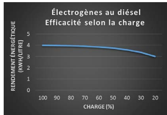
Figure 1 : Efficacité selon la charge.
