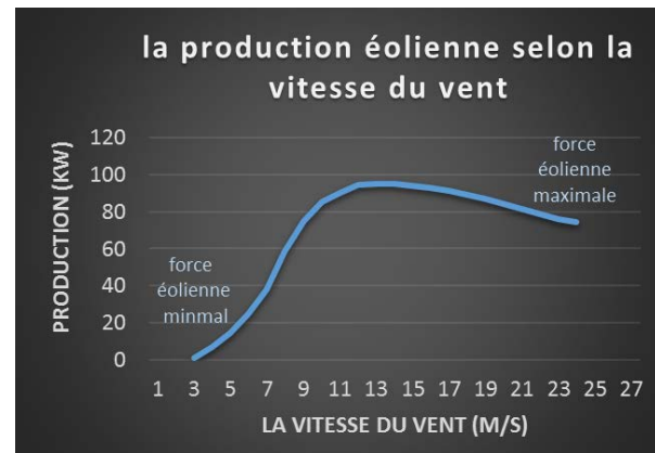
Figure 4 : Illustration de la production éolienne selon la vitesse du vent.
