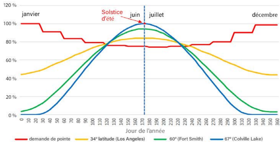
Figure 3 : Demande de pointe et ensoleillement — Fourni par la NTPC.
