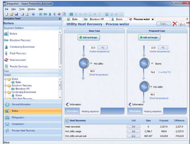
Comparaison de la récupération de chaleur des systèmes utilitaires pour une situation existante et une situation modifiée
