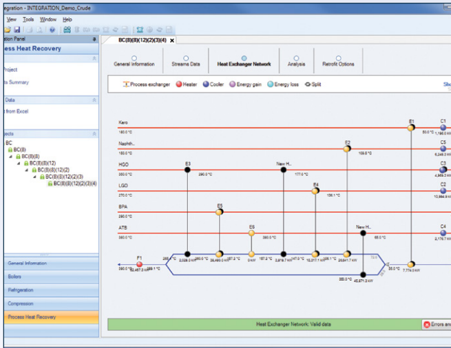
Réseau d'échangeurs de chaleur optimisé après plusieurs changements pour augmenter la récupération de chaleur
