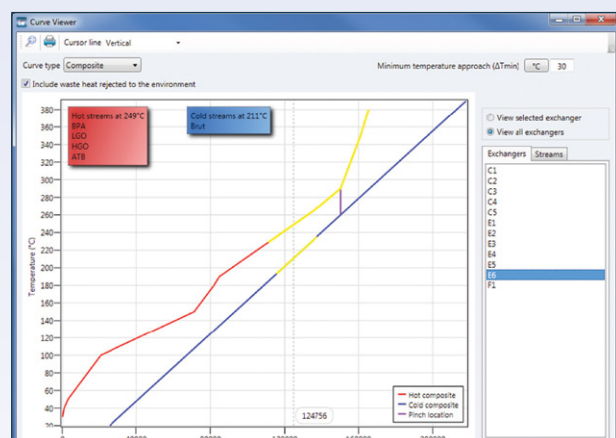
Courbes composites interactives, illustrant les besoins de chauffage et de refroidissement du procédé, ainsi que les échanges de chaleur existants
