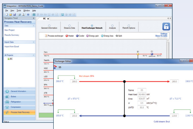
Réseau d'échangeurs de chaleur (grille du réseau) et éditeur pour un échangeur individuel
