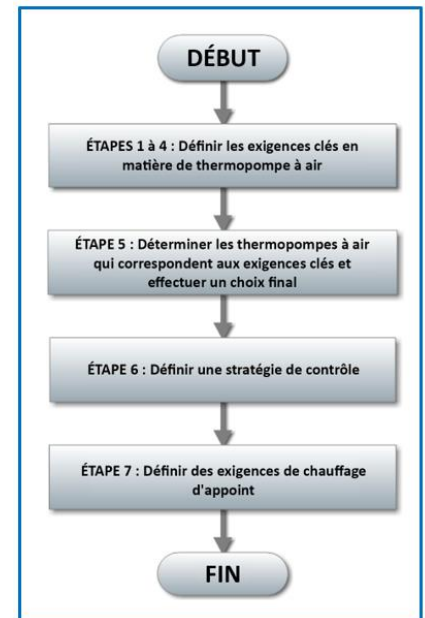
Figure 1: Aperçu du processus de dimensionnement et de sélection des thermopompes à air
