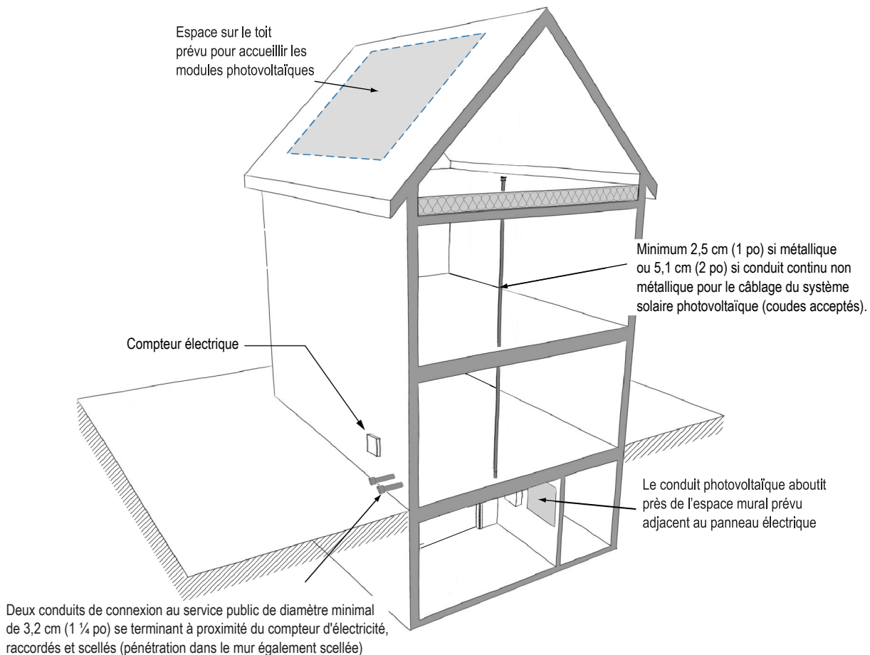
Figure 6 : Spécifications du conduit photovoltaïque et conduits de connexion au service public
