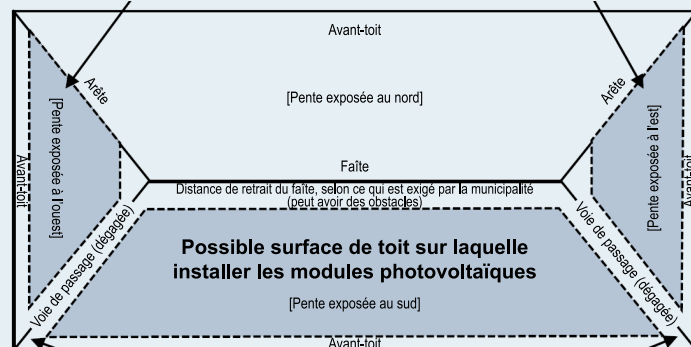
Des voies de passage dégagées le long des arêtes du toit, selon ce qui est exigé par la municipalité, lorsque des modules photovoltaïques sont installés sur des pentes adjacentes Les zones ombrées représentent les possibles surfaces du toit sur lesquelles installer des modules photovoltaïques
