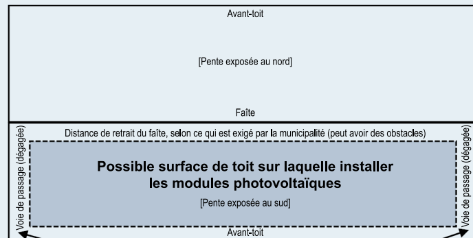
Deux voies de passage dégagées, selon ce qui est exigé par la municipalité, sur chaque pente du toit où des modules photovoltaïques sont installés Les zones ombrées représentent les possibles surfaces du toit sur lesquelles installer des modules photovoltaïques
