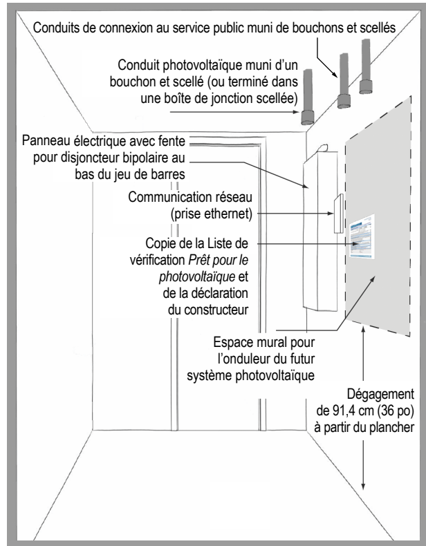
Figure 8 : Espace mural, communication réseau, prévu aboutissement du conduit photovoltaïque et conduits de connexion au service public adjacent au panneau électrique
