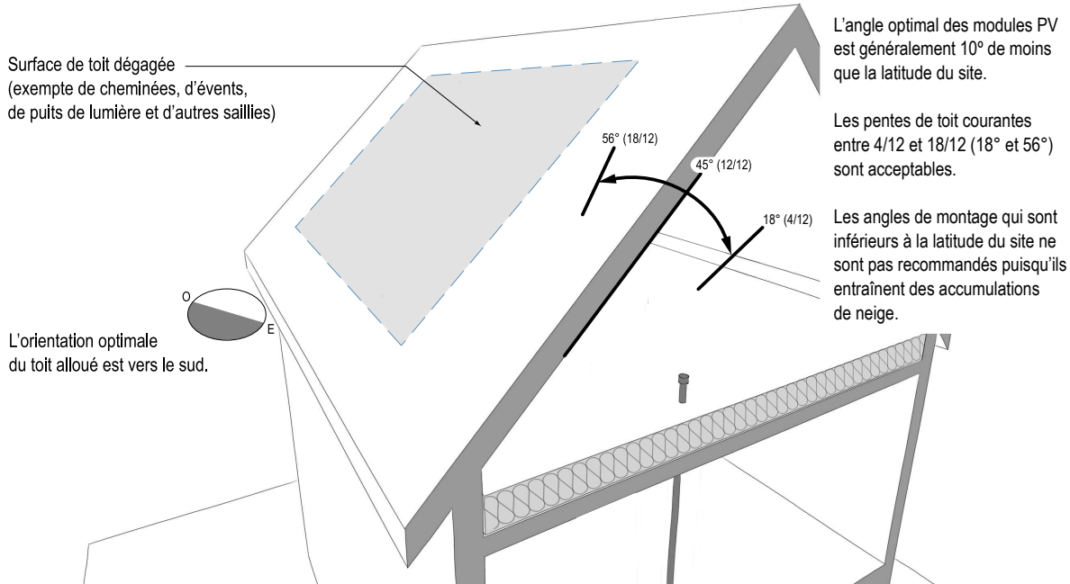
Figure 1 : Espace sur le toit, orientation et angle de montage des modules photovoltaïques
